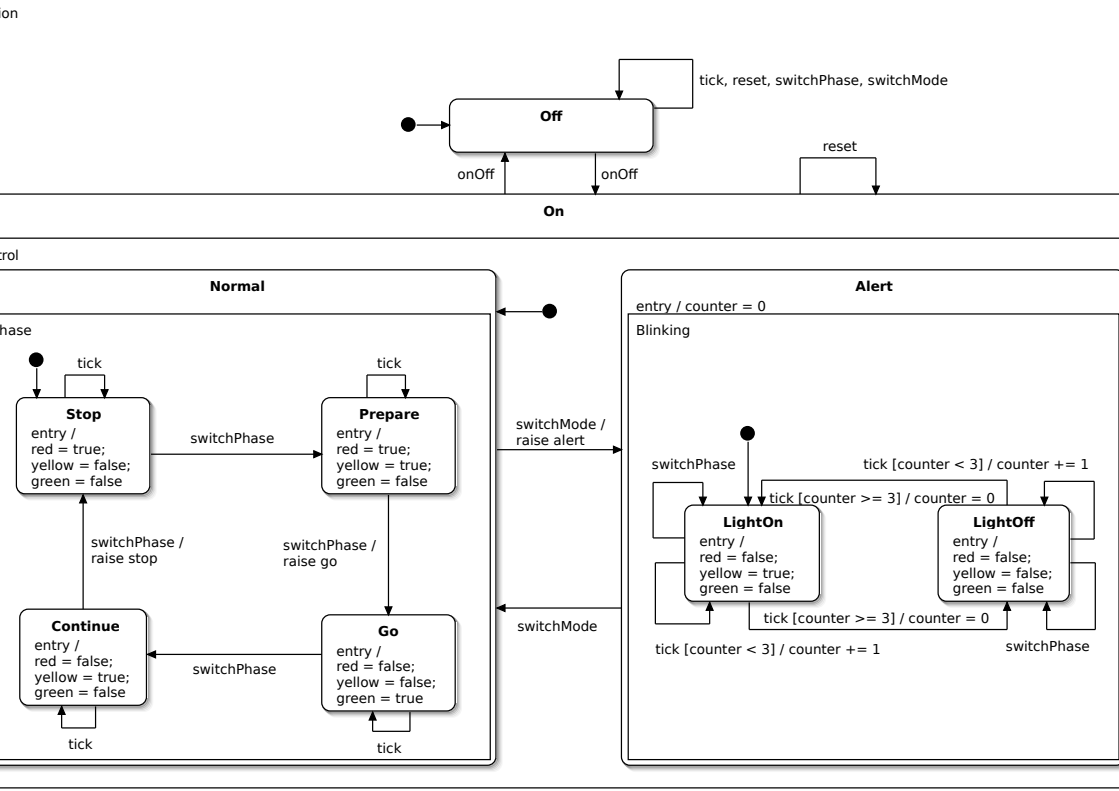
9. ábra. Fények állapotának modellezése változókkal
