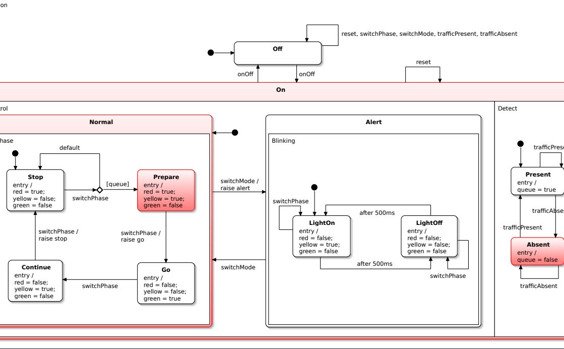
13. ábra. Ortogonális állapot aktuális állapotként
