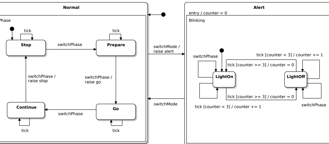
8. ábra. Villogó jelzés számlálóval
