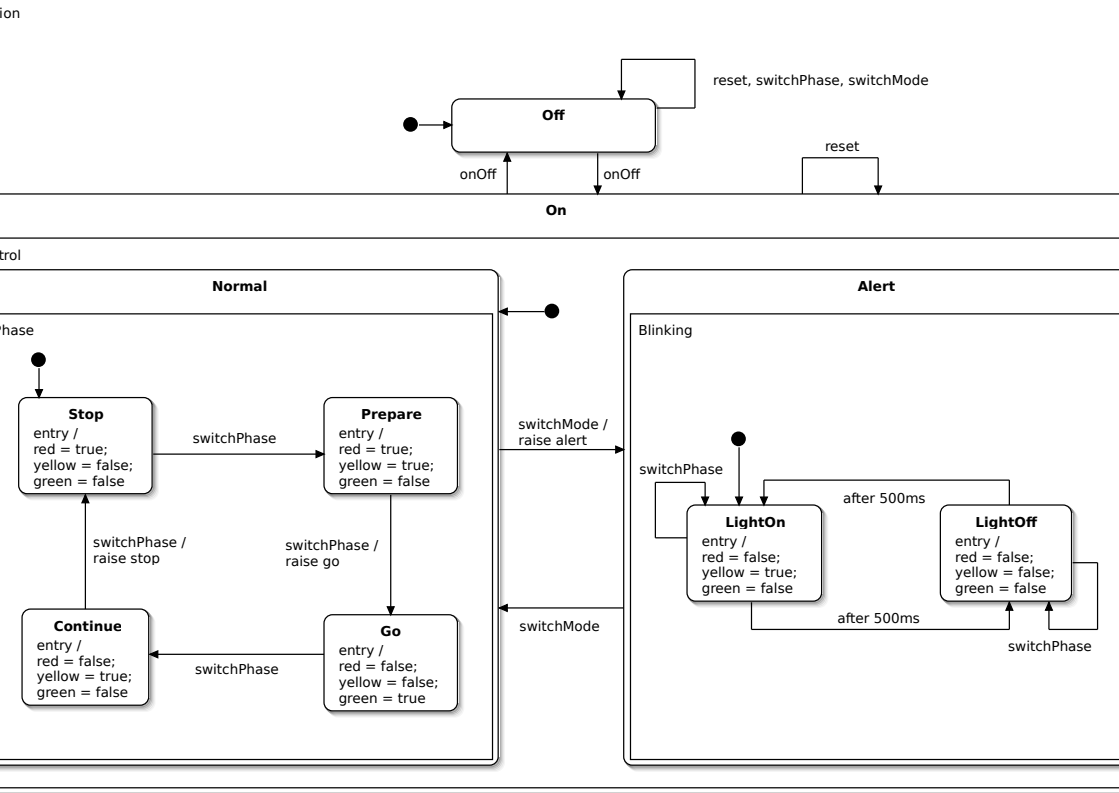
10. ábra. Villogó jelzés időzítéssel
