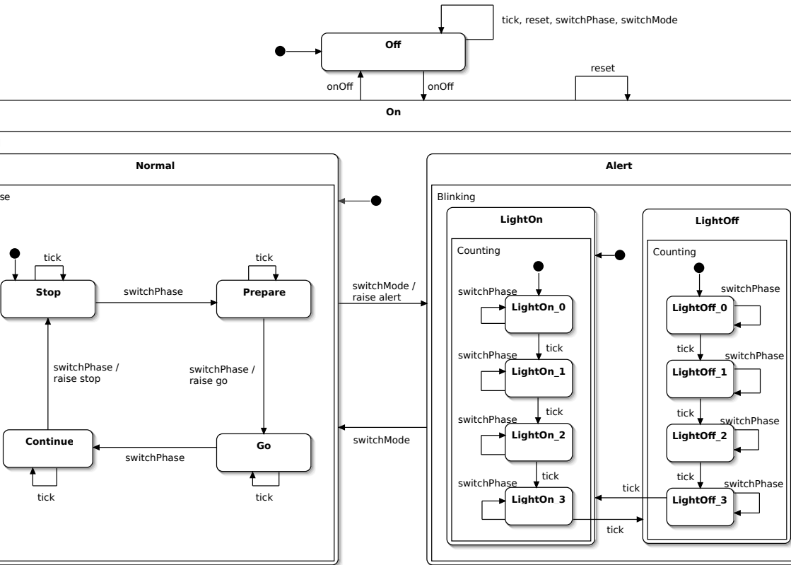
7. ábra. Villogó jelzés külső órával ☠
