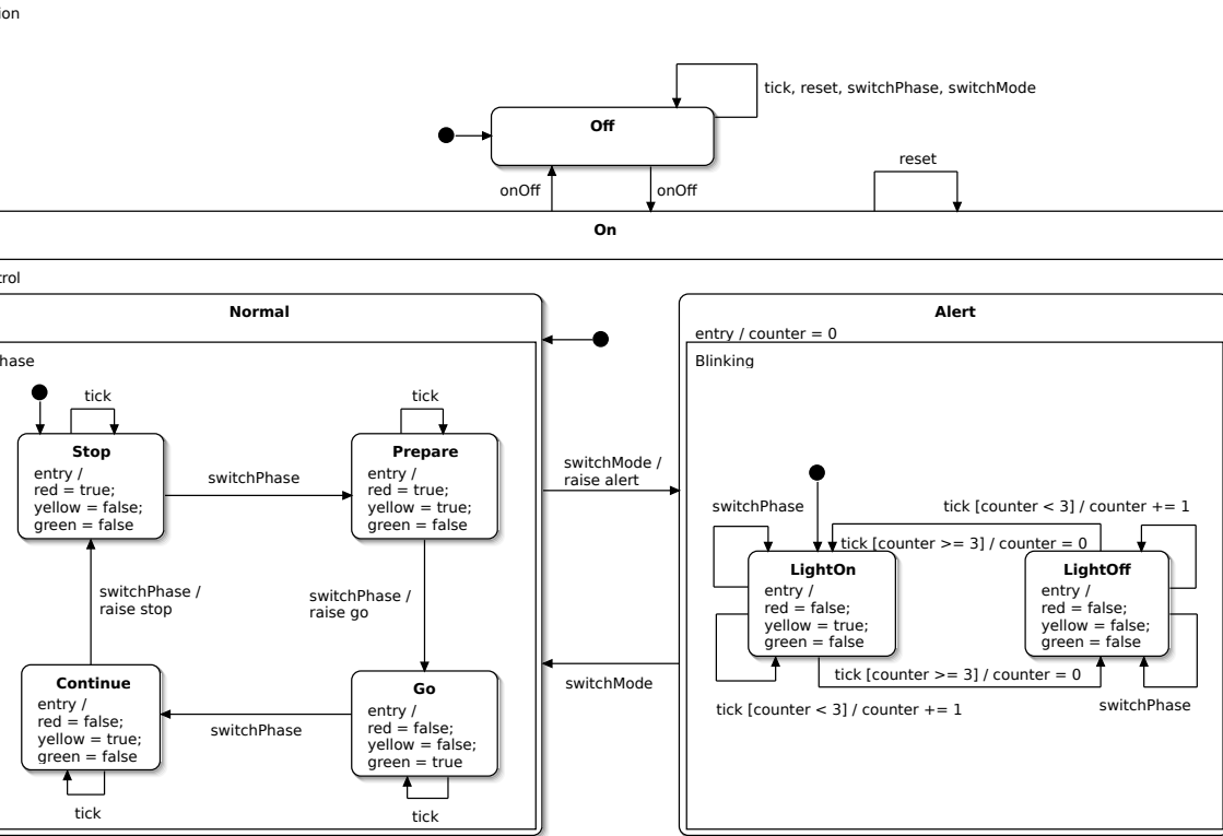
4.9. ábra. Fények állapotának modellezése változókkal
