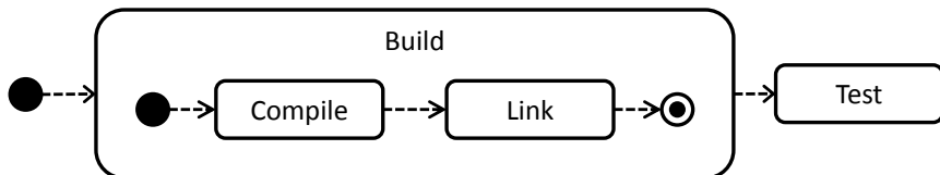
5.15. ábra. Hierarchia grafikus szintaxisa
