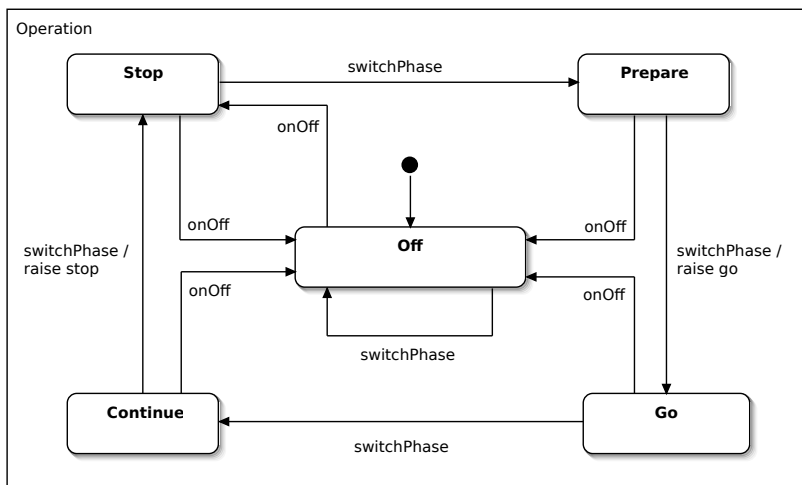
4.1. ábra. Jelzőlámpa egyszerű állapotgépe
