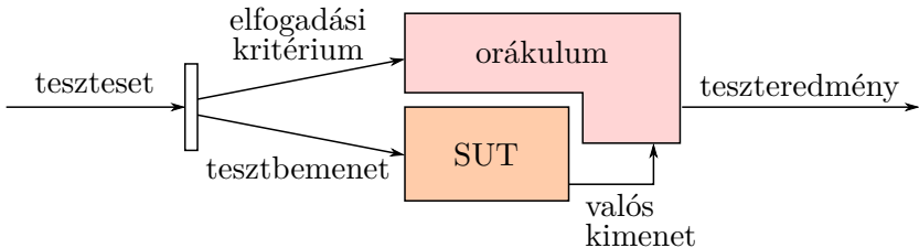
7.5. ábra. A tesztelés általános sémája
