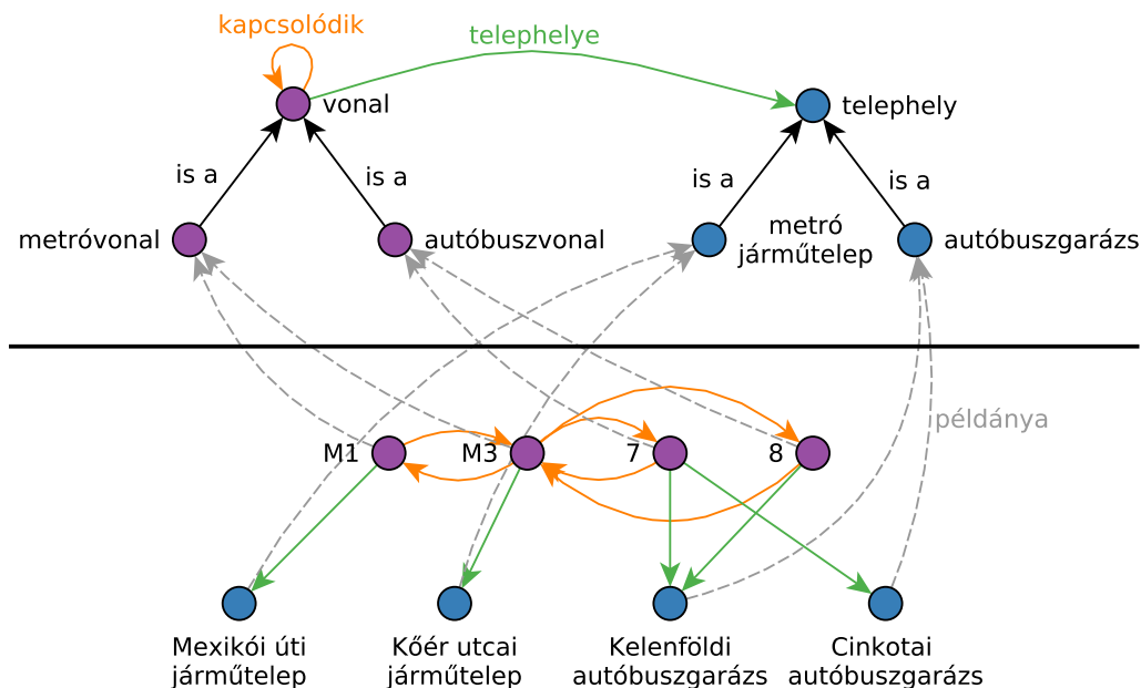
3.12. ábra. Közlekedési vonalak és telephelyek példánymodellje és (részleges) metamodellje egy gráfon ábrázolva
