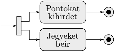
7.4. ábra. Folyamatmodell két termináló csomóponttal
