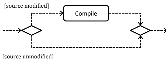
5.9. ábra. Elágazás üres ággal
