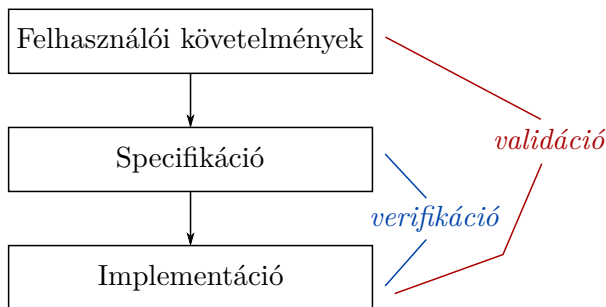
7.2. ábra. A verifikáció és a validáció közti különbség illusztrációja
