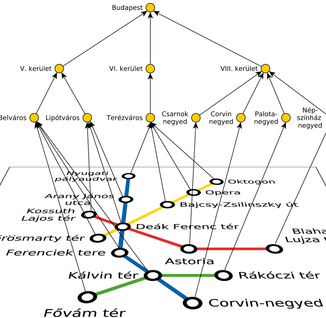
3.6. ábra. Budapest metróhálózata és a városrészek, kerületek hierarchiája
