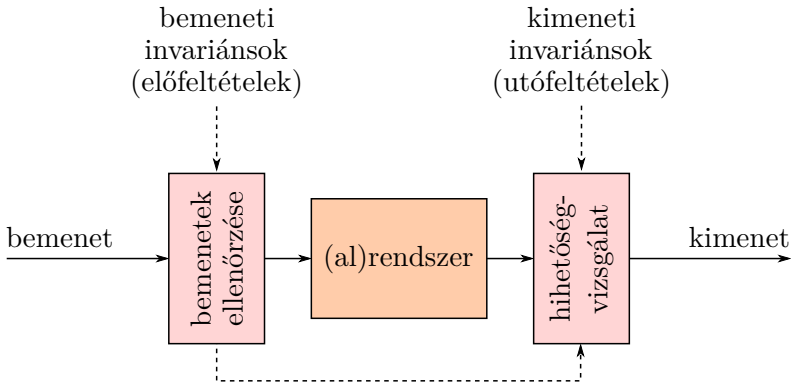
7.7. ábra. A monitorozás általános elrendezése
