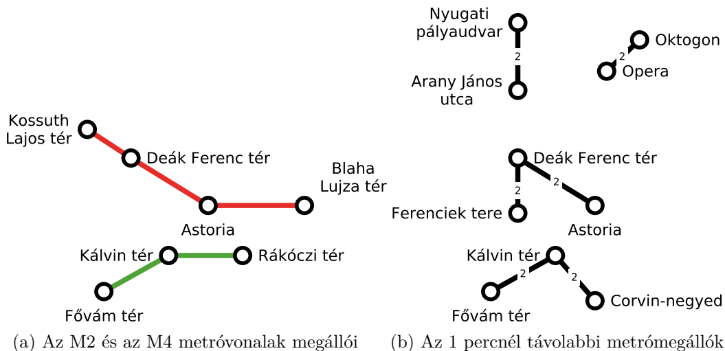
3.14. ábra. Szűrések a metróhálózatot tartalmazó gráfon
