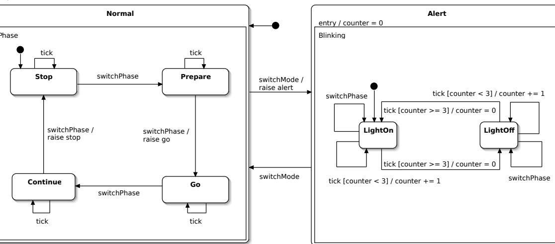
4.8. ábra. Villogó jelzés számlálóval
