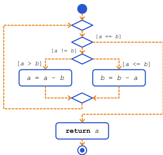
5.17. ábra. A ciklomatikus komplexitás fogalmai. E : élek (narancssárga), N csomópontok (kék)
