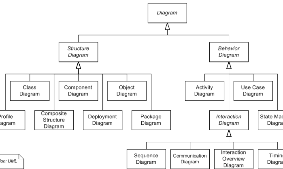
3.17. ábra. UML diagramok típusai és a közöttük lévő viszony osztálydiagramként ábrázolva [33]
