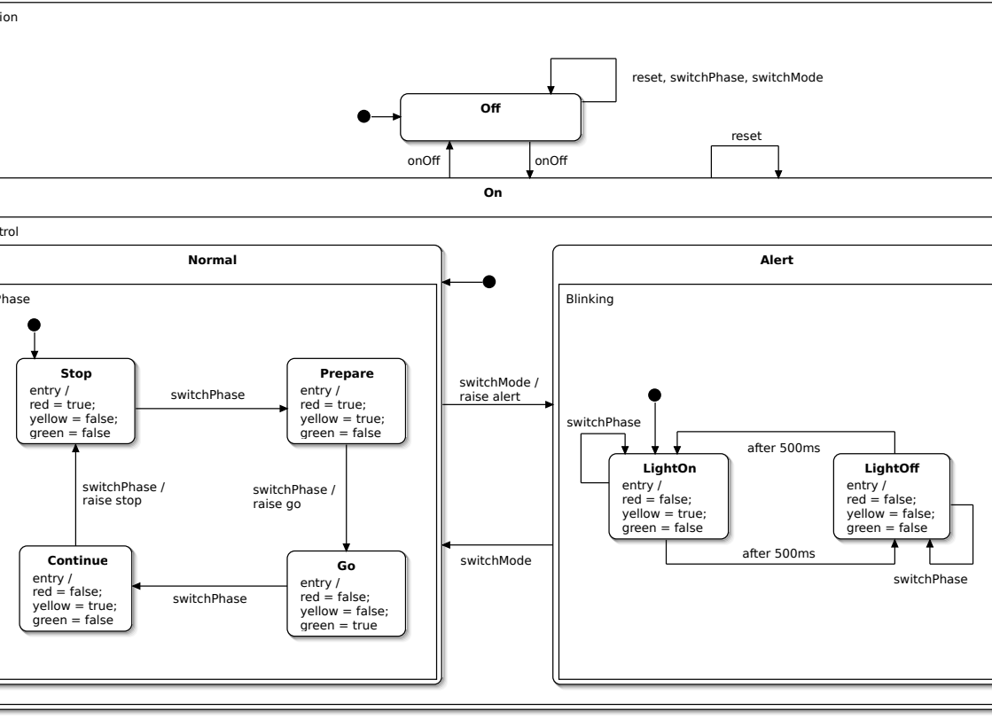
4.10. ábra. Villogó jelzés időzítéssel
