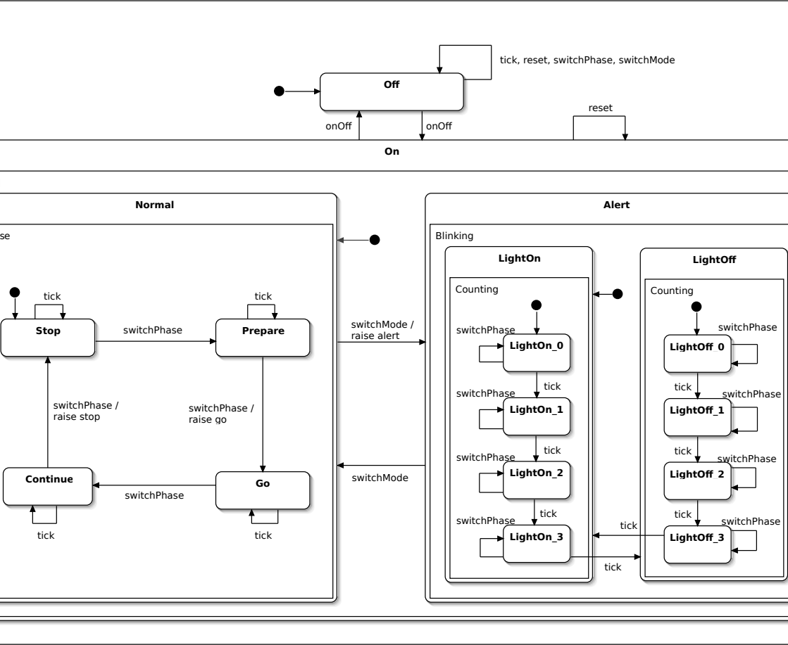
4.7. ábra. Villogó jelzés külső órával ☠
