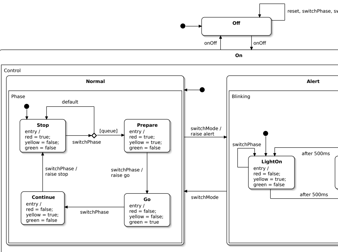
4.12. ábra. Járműérzékelős jelzőlámpa állapotgépe ortogonális
