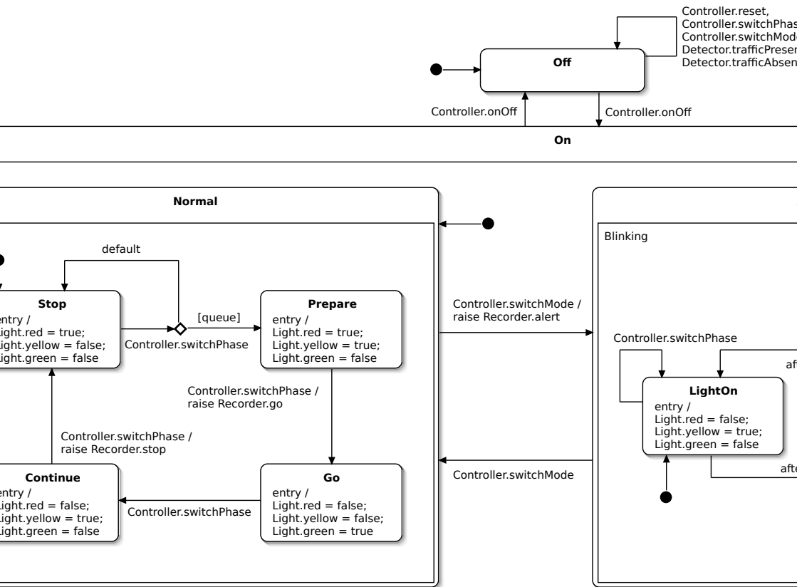
4.14. ábra. A jelzőlámpa modellje interfészekkel
